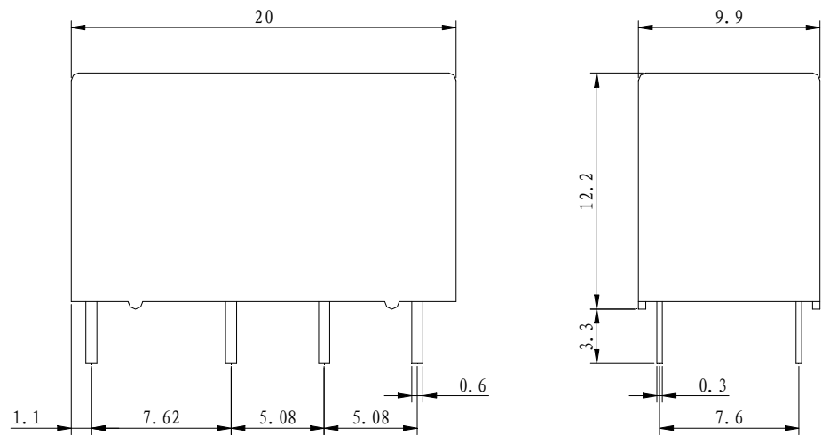
Outline Dimension 外形尺寸(mm)
