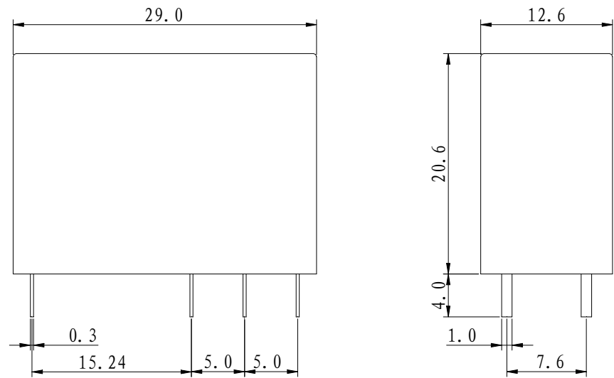
Outline Dimension 外形尺寸 (mm)
