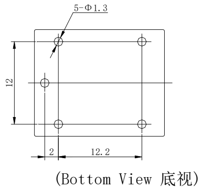
PC Board layout 安装图
