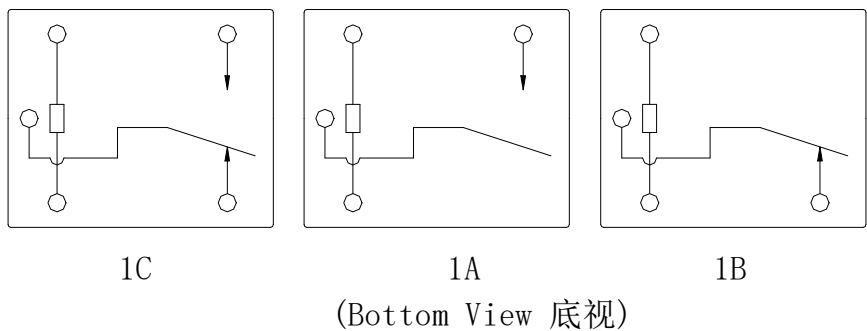
Wiring Diagram 接线图
